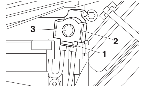
1. Fusible de reserva 2. Soporte del relé de arranque 3. Relé de arranque
