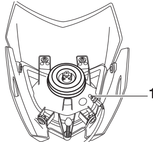
1. Bombilla de la luz de posición delantera
